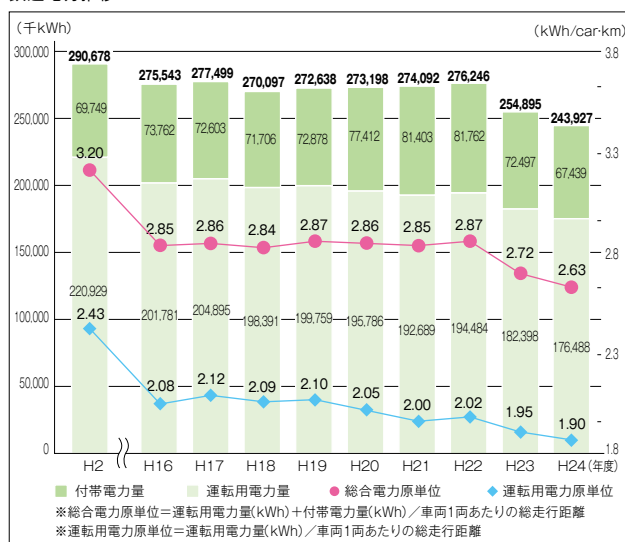
鉄道電力推移
