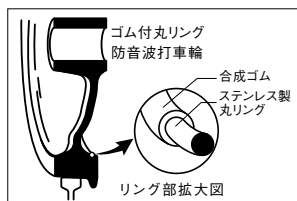
防音車輪の仕組み
