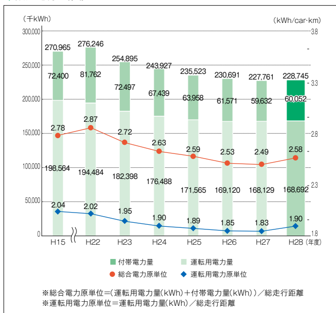
◆鉄道電力の推移
